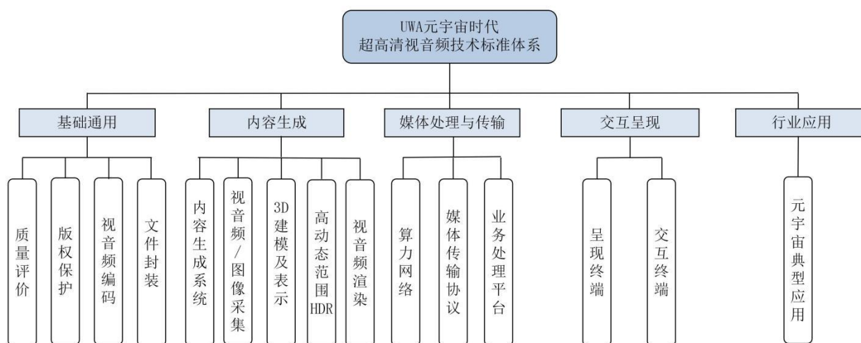
图 11 UWA 元宇宙时代超高清视音频技术体系框架
